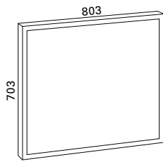
EVO 80X70 • mitat L803 x K703 x S38 mm
