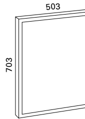
EVO 50X70 • mitat L503 x K703 x S38 mm
