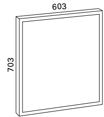
EVO 60X70 • mitat L603 x K703 x S38 mm
